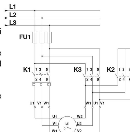
Fig. 11 Collegamenti stella triangolo
