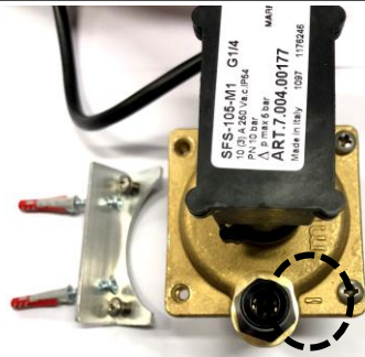
Fig.4-5 – IT- Avvitare la staffa (D) al differenziale di pressione (F) nel lato specularmente opposto a quello con il segno “-“ (cerchiato). EN- Screw the metal bracket (D) to the differential of pressure (F) in the symmetrically opposite side of the one with the “-“ sign (circled). FR- Visser le support (D) sur le différentiel de pression (F) du côté opposé à celui portant le signe “-“ (entouré). ES- Enroscar el soporte metálico (D) en el presostato diferencial (F), en el lado simétricamente opuesto a aquel con el marcador “-“ (señalado en la imagen). DE – Schrauben Sie den Bügel (D) auf der Rückseite der Seite mit dem “-“-Zeichen (eingekreist) an den Differenzdruckregler (F).
