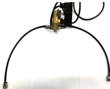
Fig.6 – IT - Tagliare in due parti uguali il tubo nero (G) ed inserirli ognuno negli attacchi rapidi precedentemente avvitati al differenziale di pressione (Fig.3) ed agganciare alle estremità gli attacchi rapidi (C) che andranno collegati nella tubazione in ingresso ed in uscita del filtro. ATTENZIONE: Il segno “+” stampato in rilievo sul differenziale di pressione indica la corrispondenza dell’ingresso dell’acqua; viceversa, il segno “-“ stampato in rilievo sul differenziale di pressione indica la corrispondenza dell’uscita dell’acqua. EN- Cut into two equal parts the black tube (G). Insert each part into the rapid connections previously screwed to the differential of pressure (Fig.3) and connect the rapid connections (C) to the opposite ends; the rapid connections (C) will be connected to the inlet and the outlet of the filter. ATTENTION: The “+” sign stamped on the differential of pressure indicates the side of the water inlet connection; conversely, the “-“ sign indicates the side of the water outlet connection. FR - Couper le tube noir (G) en deux parties égales et les insérer dans les raccords rapides précédemment vissés au différentiel de pression (Fig.3) et accrochez les raccords rapides (C) aux extrémités qui seront connectées à l’entrée et à la sortie du filtre. ATTENTION: Le signe “+” imprimé en relief sur le différentiel de pression indique la correspondance de l’entrée d’eau; inversement, le signe “-“ imprimé en relief sur le différentiel de pression indique la correspondance de la sortie d’eau. ES - Cortar en dos partes iguales la manguera (G) e insertarlas en las conexiones rápidas anteriormente enroscadas en el presostato (Fig.3) y engancharlas en las extremidades. Las conexiones rápidas van a ir conectadas a la tubería a la entrada y salida del filtro. ATENCIÓN: la marca “+” impresa en el presostato diferencial indica el lado de entrada del agua; viceversa, la marca “-“ impresa en el presostato diferencial indica el lado de salida del agua. DE – Schneiden Sie den schwarzen Schlauch (G) in zwei gleiche Teile und stecken Sie diese jeweils in die Schnellkupplungen, die zuvor an den Differenzdruckregler geschraubt wurden (Abb.3), und schließen Sie die Schnellkupplungen (C) an den Enden an, die mit den Ein- und Auslassleitungen des Filters verbunden werden. ACHTUNG: Das eingeprägte “+“-Zeichen auf dem Differenzdruckregler zeigt den Wassereingang an. Umgekehrt zeigt das eingeprägte “-“-Zeichen auf dem Differenzdruckregler den Wasserausgang an.
